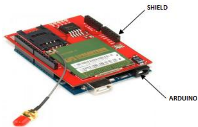
Figura 9: Acoplamento Shield x Arduino
