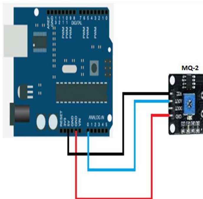
Figura 3: Detalhamento do esquema de conexão do sensor de gás e fumaça x Arduino
