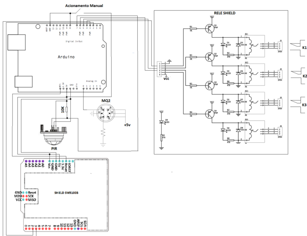
Figura 10: Diagrama geral
