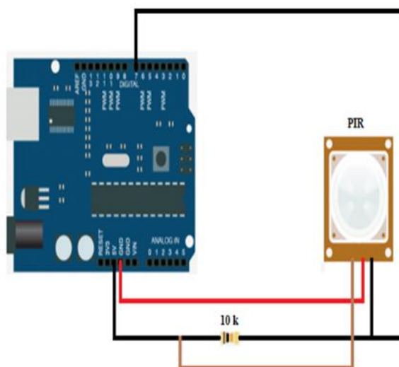
Figura 5: Detalhamento do esquema de conexão do sensor PIR x Arduino
