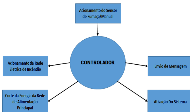
Figura 1: Fluxograma do Sistema de Combate ao Incêndio.
