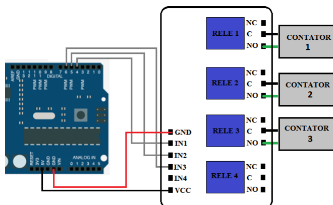
Figura 7: Detalhamento do esquema de conexão do RelShield x Arduino
