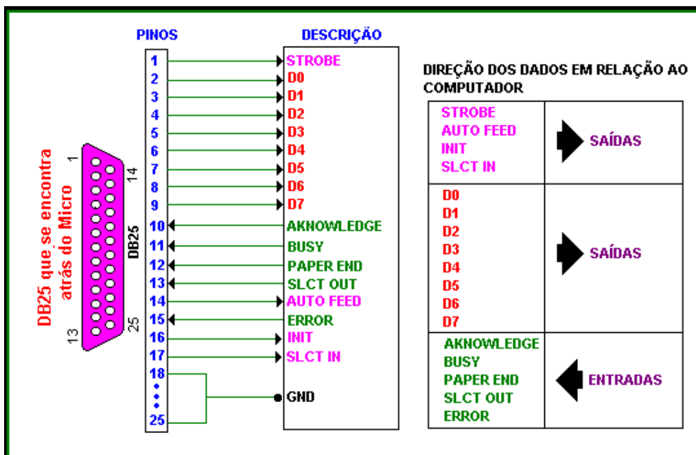
Figura 4 - Esquema de Funcionamento do DB25
